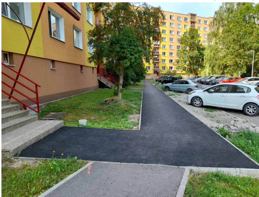
Obrázok č. 53 Rekonštrukcia rozvodov ÚK a TV – okruh kotolne Mier 1, vetva sever, časť 3
